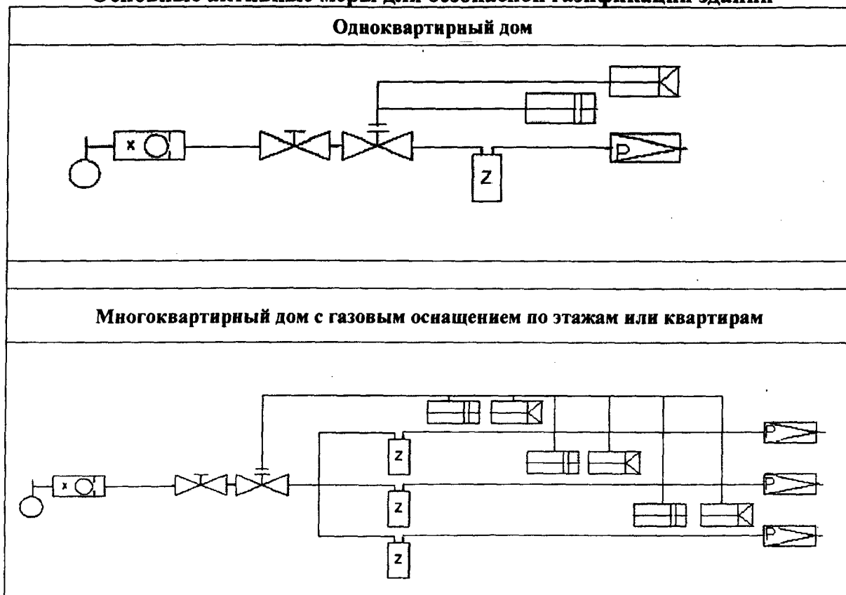
Рисунок Д.1 — Активные меры безопасности при давлении в наружном газопроводе свыше 0,0025 МПа до 0,005 МПа включительно и приборы, регулирующие давление газа
