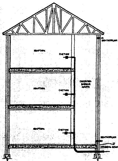
Рисунок Г.2 — Газопровод в вентилируемой шахте
